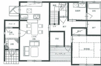
設計図
